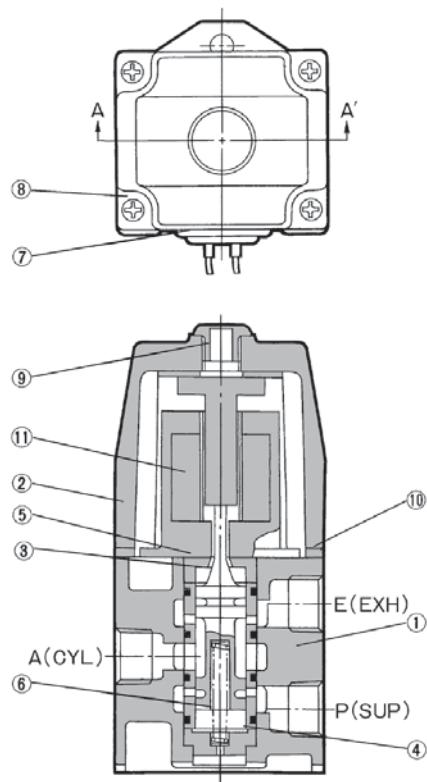
A-A' 断面图
