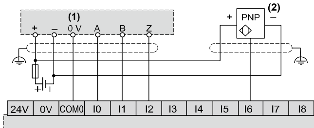
(1) 带有索引的双相编码器 (2) PNP 传感器
