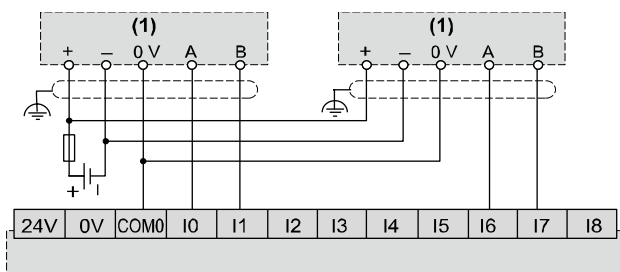
(1) 不带索引的双相编码器
