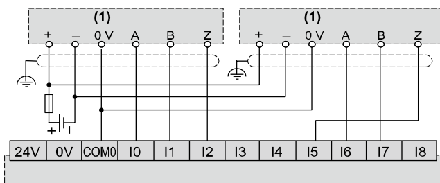
(1) 带有索引的双相编码器
