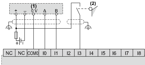
(1) 不带索引的双相编码器 (2) 限位开关
