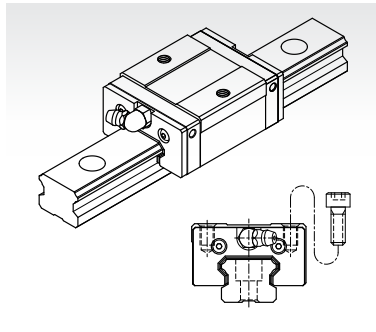
MSB-TS 型
