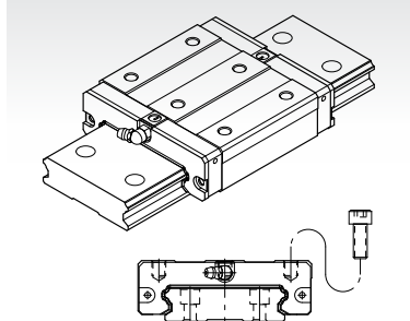
MSG-S型
