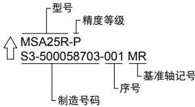
滑块的标记
