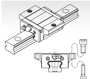
MSB-TE 型
