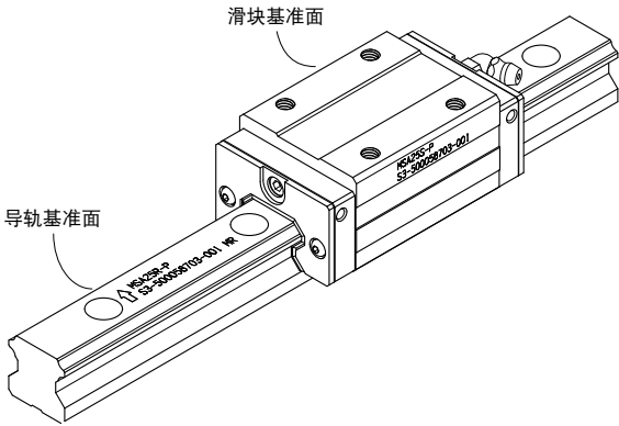
导轨的标记
