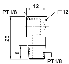
OL-C型
