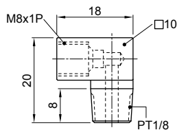
OL-D型
