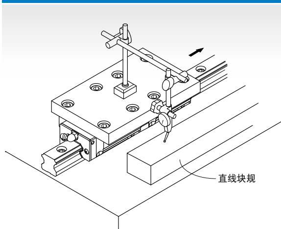
千分量表测定法
