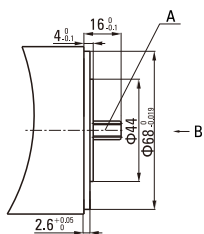
电机配合方案 Motor Matching Scheme
