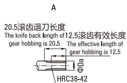
电机配合方案 Motor Matching Scheme
