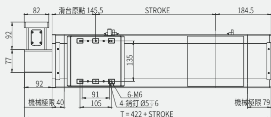
AIMTW178-LB-DB 馬達左側直接安裝 motor leftside direct installed
