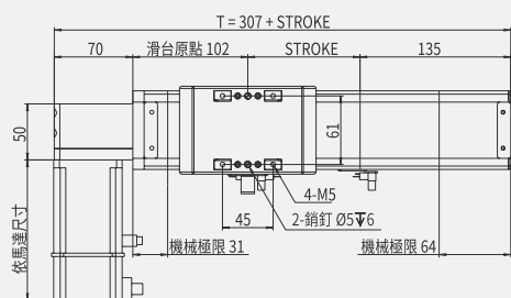
AIMTW70-1P-RM 馬達右側插軸安裝 motor rightside hollow shaft installed
