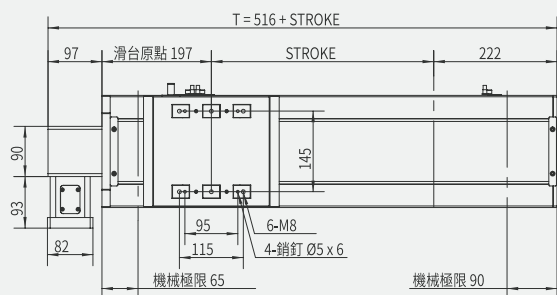
AIMTW202-4P-LF-DF 馬達右側直接安裝 motor rightside direct installed
