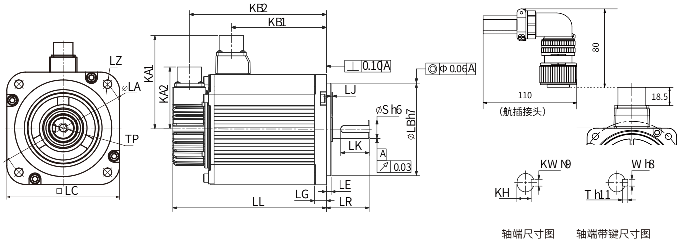
MS1H3/ISMH3（Vn=1500rpm，Vmax=3000rpm）系列外形尺寸图（单位：mm）
