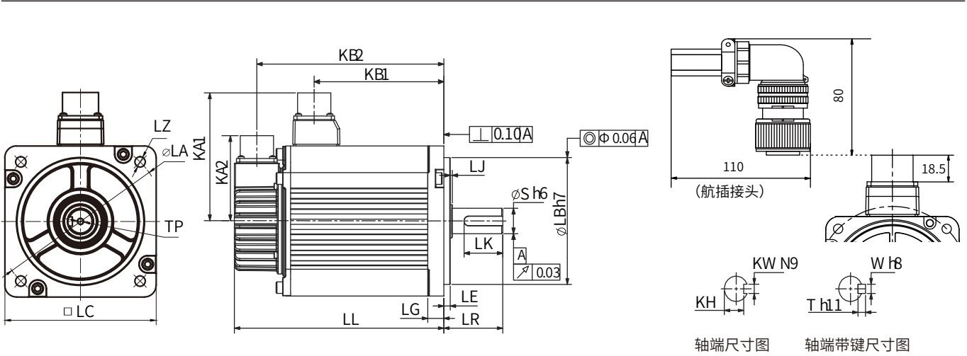
ISMH2（Vn=3000rpm，Vmax=6000/5000rpm）系列外形尺寸图（单位：mm）
