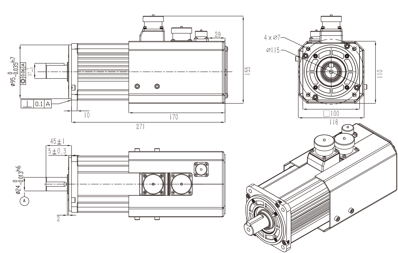
MS1V2 电机外形尺寸图（单位：mm）
