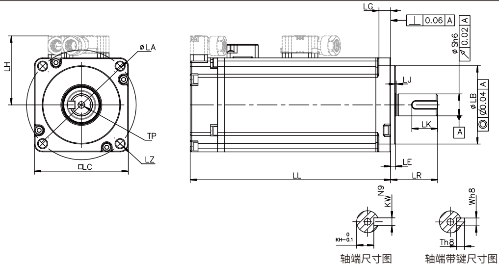
MS1H4系列外形尺寸图（单位：mm）
