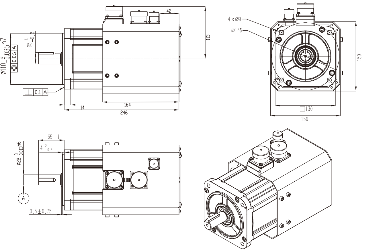
MS1V3 电机外形尺寸图（单位：mm）
