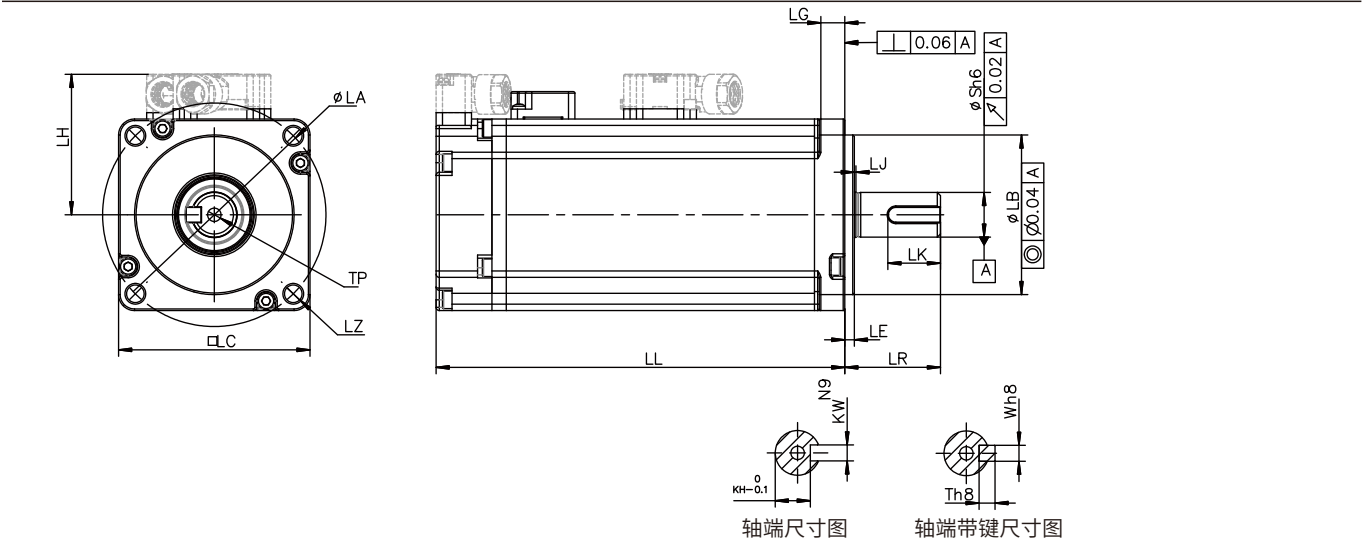
MS1H1系列外形尺寸图（单位：mm）
