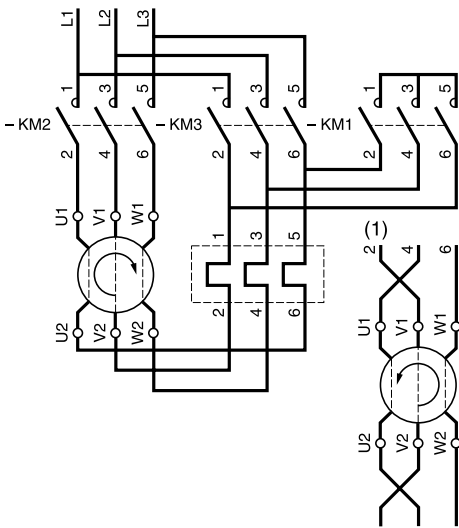
3 x LC1D09 到 D95 机械互锁在 KM3 和 KM1
