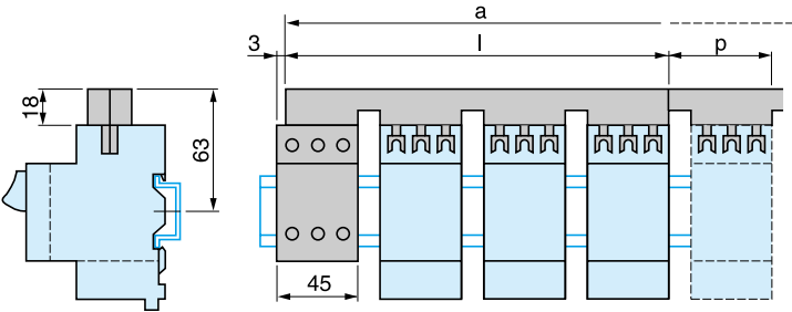
母排 GV2G●●● 带接线端子模块 GV1G09
