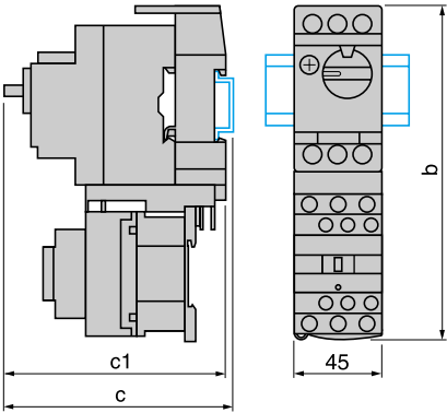
用于组合 GV2PM + D 型接触器
