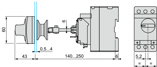
安装适用于 GV2PM 的加长操作手柄 GV2APN01 或 GV2APN02
