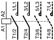
LC1D205 至 D245 ( 线圈 LX9F ~ )
