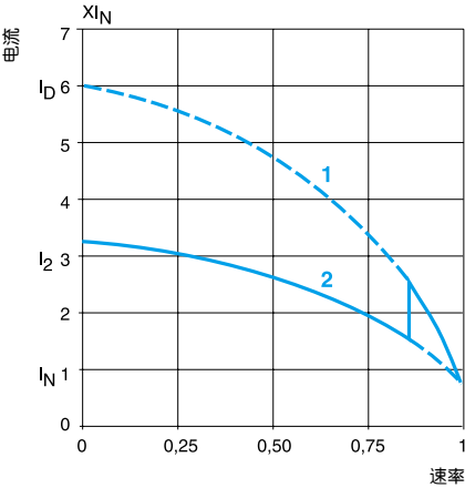
1 直接开关电流 2 带有自耦变压器的电流
