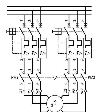
2 电源 GV2ME, GV2PM
