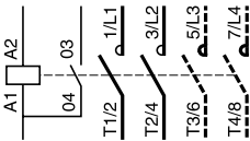
LC1D205 至 D620 ( 线圈 LX1F ~ )
