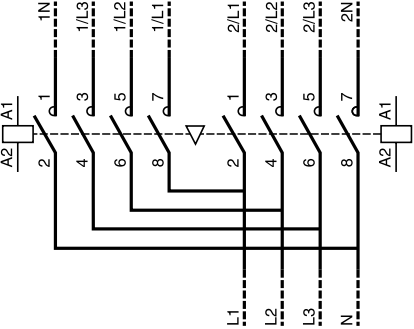
配电用的电源转换接触器组，水平安装 2 x LC1D
