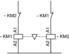
可逆接触器的电气互锁装置，装有： 机械互锁装置 不带集成电气触点 LA9F●●●
