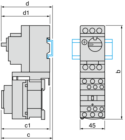
用于组合 GV2PM + D 型接触器
