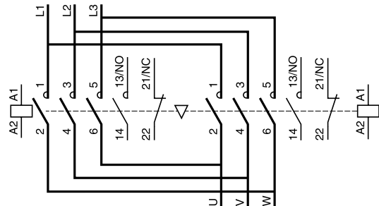
电源切换接触器组，水平安装 LC2DT20...DT40
