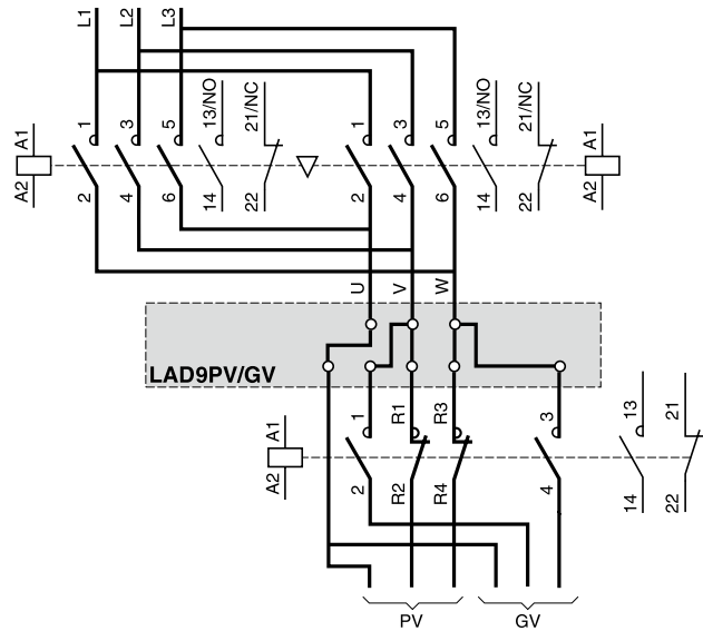
低速 / 高速配线组件、螺钉夹紧端子
