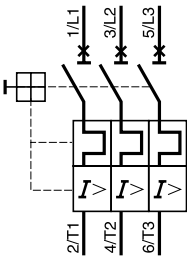
限流器 GV1L3
