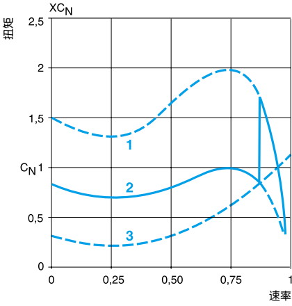
1 直接电动机扭矩 2 带有自耦变压器的扭矩 3 机器的阻性扭矩
