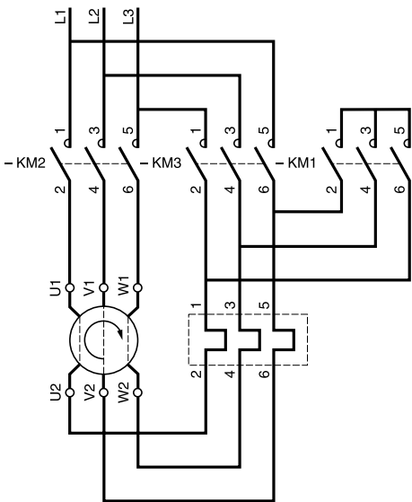
3 x LC1D115 到 D170
