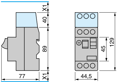
GV2ME + GV1L3 (限流器)
