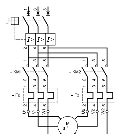
部分绕组电动机 GV2LE
