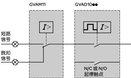
故障信号触点和短路信号触点的应用
