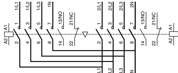
可逆接触器的电气互锁装置，安装了 集成有电气触点的机械互锁装置 LA9D●●●02
