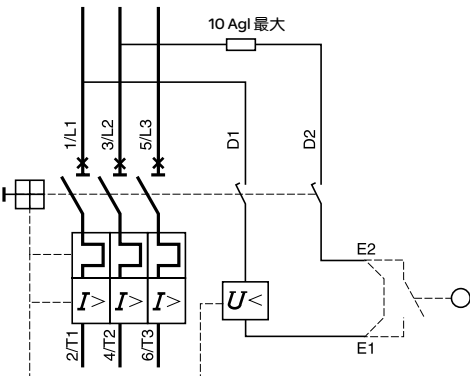
在危险设备上的欠压脱扣保护接线方式 (符合 INRS), 仅适用于 GV2ME
