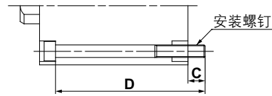
安装螺钉图
