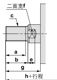
杆端 外螺纹的场合
