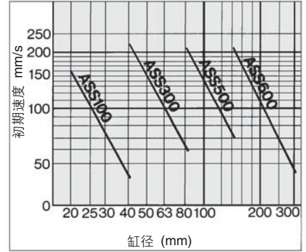
排气节流控制の場合
