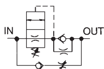
排气节流控制型
