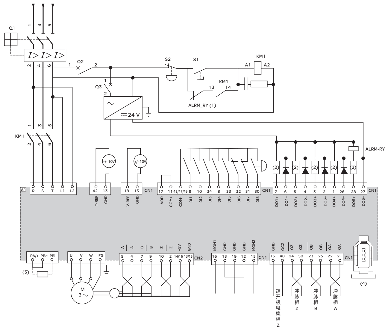
转矩控制模式接线图 LXM 23CU●●M3X
