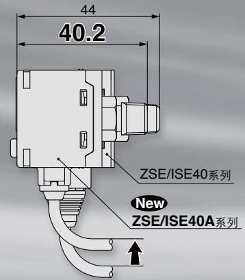
面板安装
