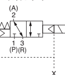
外部先导式
