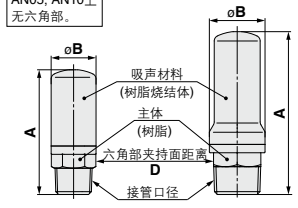
尺寸表 (mm)
